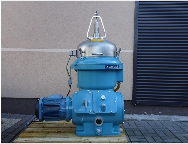
Alfa Laval WSPX 207 TGP-74 Separator
